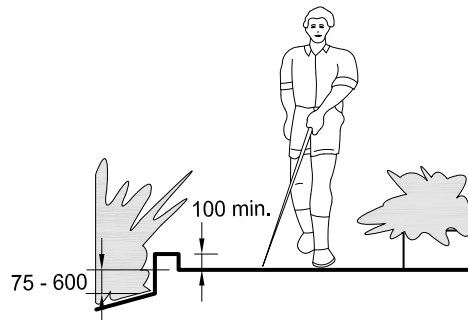
Figure 4.1.4.4: Edge Protection
